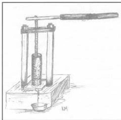
Oliepers
